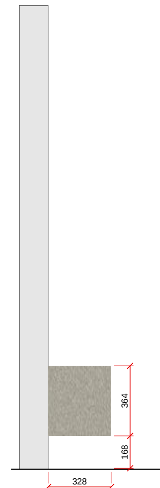
VISTA C - LATERAL - ESC. 1:20
