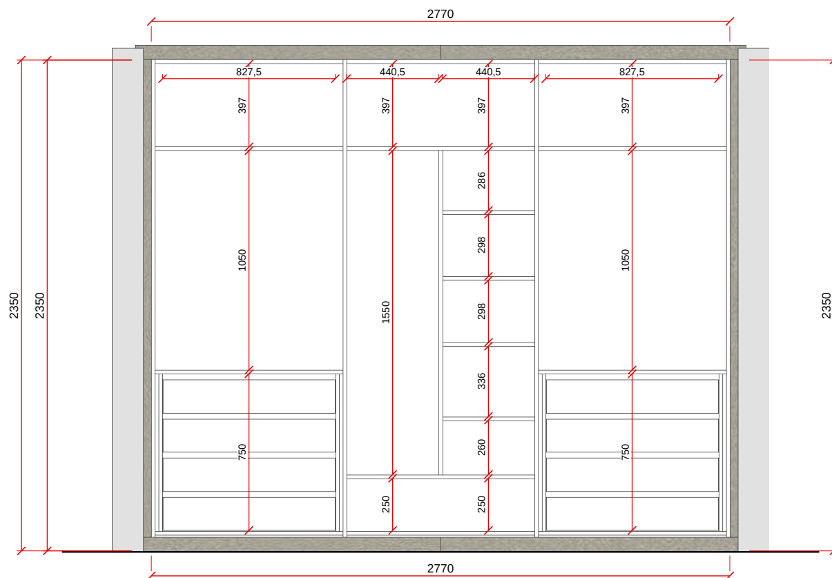
VISTA B - ESC. 1:25
