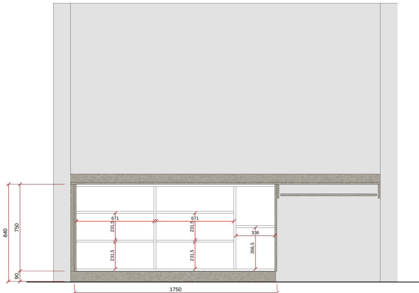
VISTA A - ESC. 1:20
