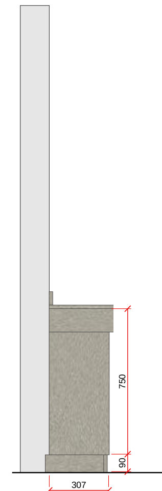
VISTA A - LATERAL - ESC. 1:20
