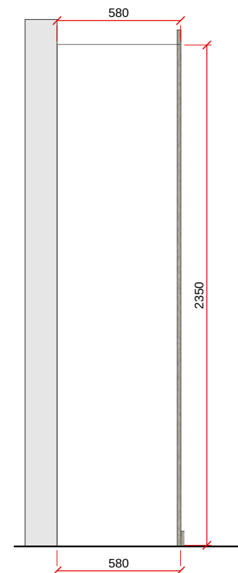
VISTA B - LATERAL - ESC. 1:25
